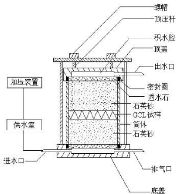
图 B1 南 55 型渗透仪装置
