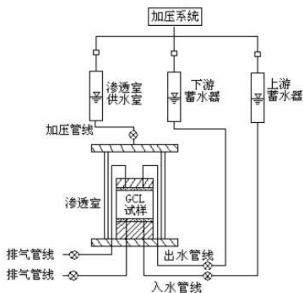
图 A1 渗透系数测定装置
