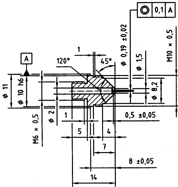
b) Gas jet
